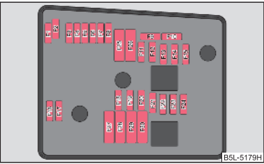
Изобр. 186 Схематическое представление коробки предохранителей в подкапотном пространстве – исполнение 2
