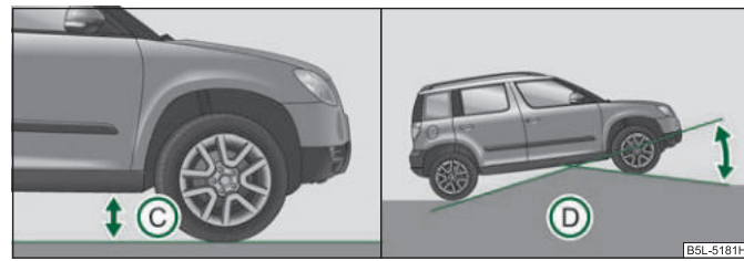
Изобр. 156 Дорожный просвет / продольный угол проходимости
