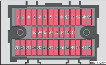
Изобр. 187 Схематическое представление коробки предохранителей в панели приборов
