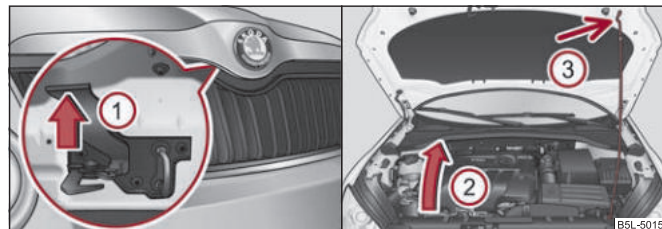
Изобр. 13 Решетка радиатора: Рукоятка фиксатора / фиксация капота двигателя опорой
