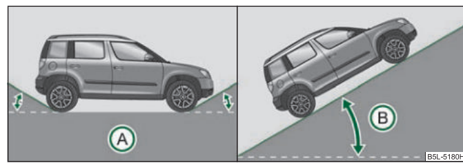
Изобр. 155 Угол наклона / угол подъема
