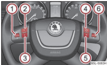
Изобр. 118 Многофункциональное рулевое колесо: кнопки управления
