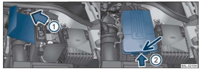
Изобр. 167 Подкапотное пространство: полиэфирный чехол аккумуляторной батареи / пластиковый чехол аккумуляторной батареи
